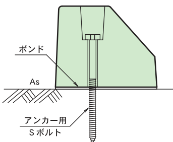
アスファルト舗装タイプ
