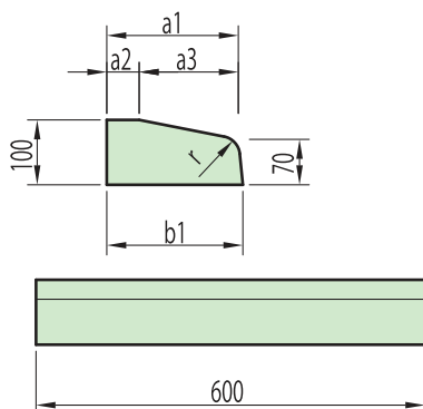
片面歩車道境界ブロック 切下げ平
