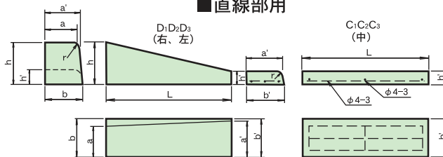
歩車道境界歩行者横断用ブロック (1本下り)
