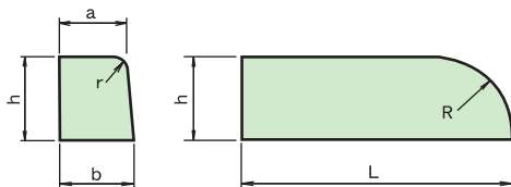
●歩車道境界端末ブロック
