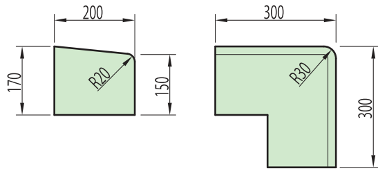
片面歩車道境界ブロックA 外コーナー
