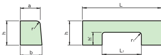
●歩車道境界水抜用ブロック
