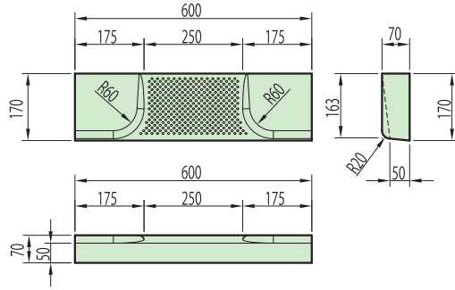
歩車道タイプ
