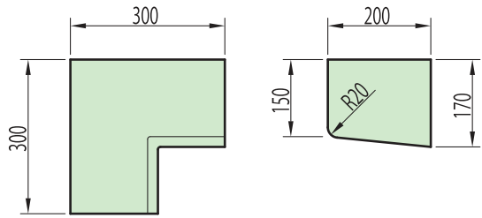
片面歩車道境界ブロックA 内コーナー
