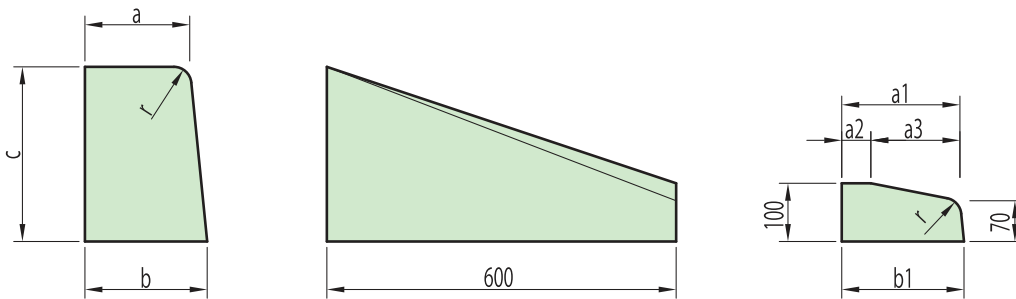
片面歩車道境界ブロック 切下げ斜
