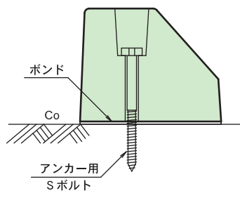
コンクリート舗装タイプ
