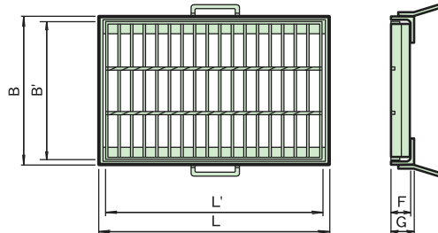
■車道用 (T-25)
