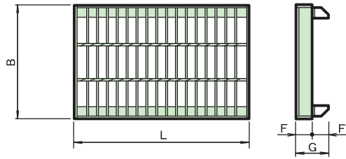
■車道用 (T-25)
