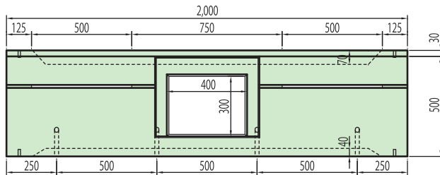
2種(管理用開口部付)：平面図
