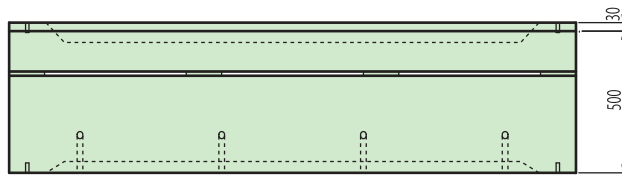
1種：平面図
