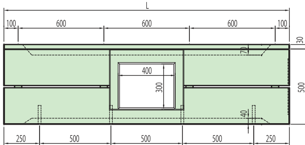
2種(管理用開口部付)：平面図
