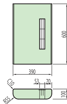
(網付) 参考重量 53 kg
