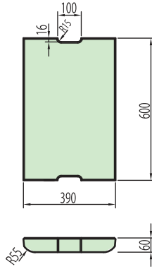
(手掛付) 参考重量 56 kg
