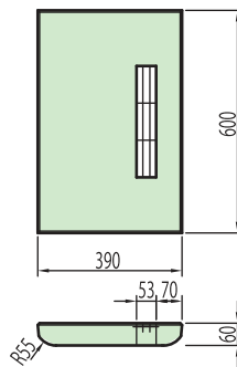
(網付) 参考重量 53 kg
