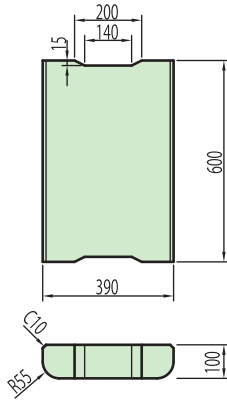
(手掛付) 参考重量 56 kg
