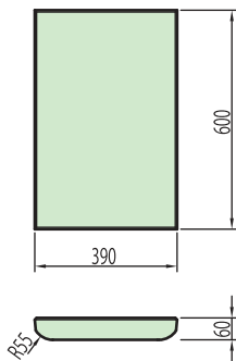
(普通) 参考重量 57 kg
