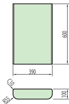
(普通) 参考重量 57 kg
