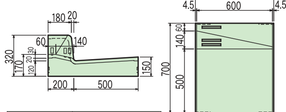
国交省L型II型MDB-1 乗入部斜
