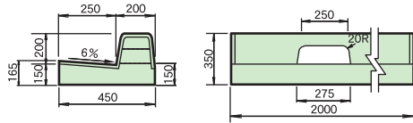
標準型 FS-C水抜き
