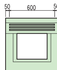
国交省L型II型MDB-1 乗入部縁塊
