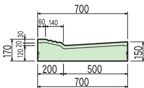
国交省L型II型MDB-1 乗入部 (L=2m)
