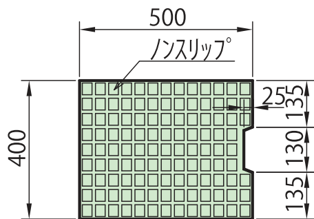
歩道用コンクリート蓋 300用
