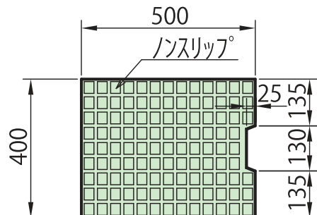
車道用コンクリート蓋 300用
