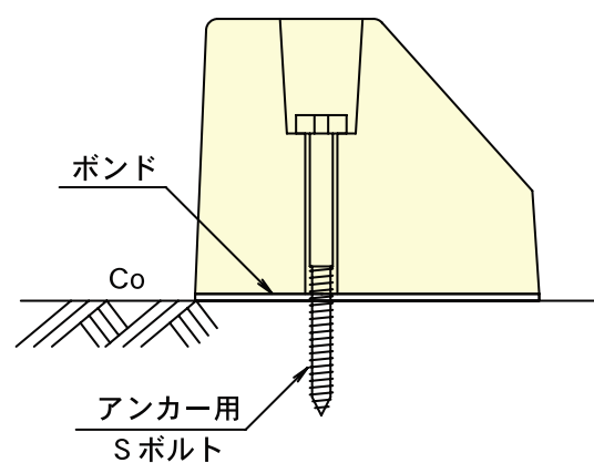
コンクリート舗装タイプ
