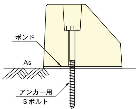
アスファルト舗装タイプ
