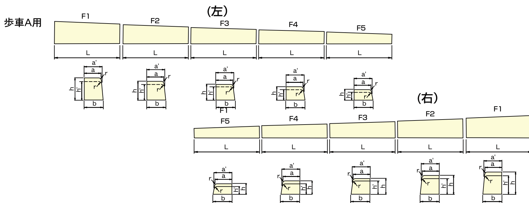
歩車道境界歩行者横断用ブロック
