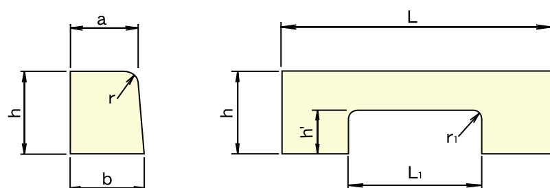
●歩車道境界水抜用ブロック
