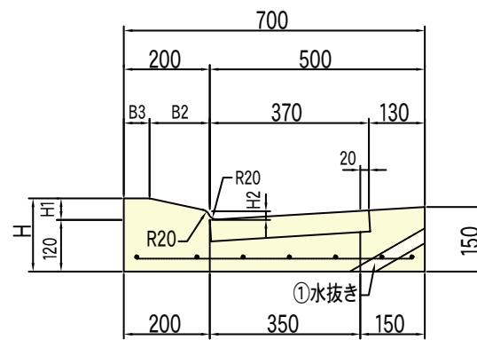
平縁塊側面図
