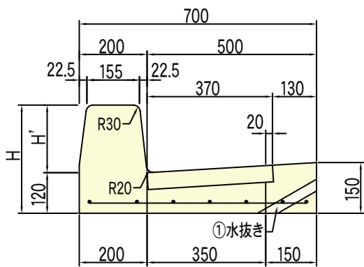
基本縁塊側面図
