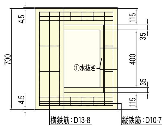
配筋図
