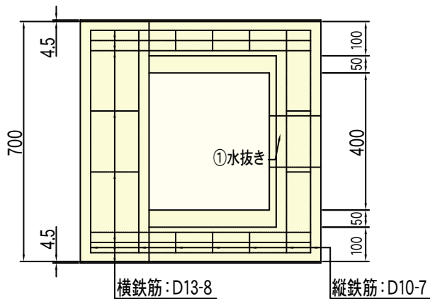
配筋図
