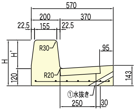
基本縁塊側面図
