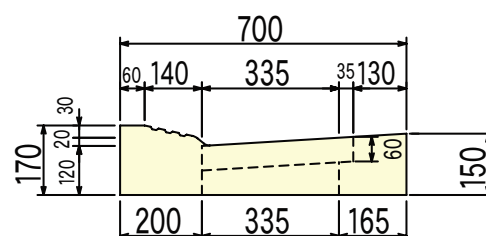
国交省L型II型MDB-1 乗入部縁塊
