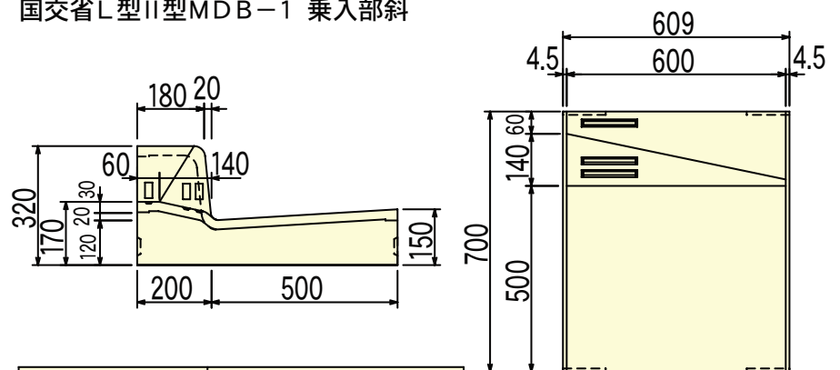
国交省L型II型MDB-1 乗入部斜
