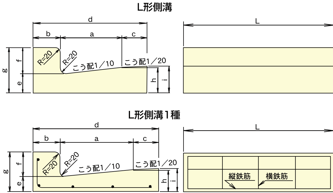
L形側溝
