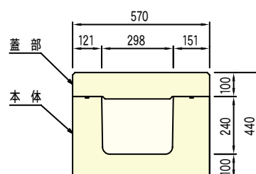
■ 300×240 (組合せ図)
