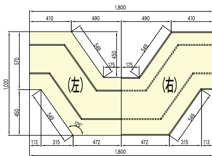
■ 蓋部 (左右2分割) W=166kg/枚
