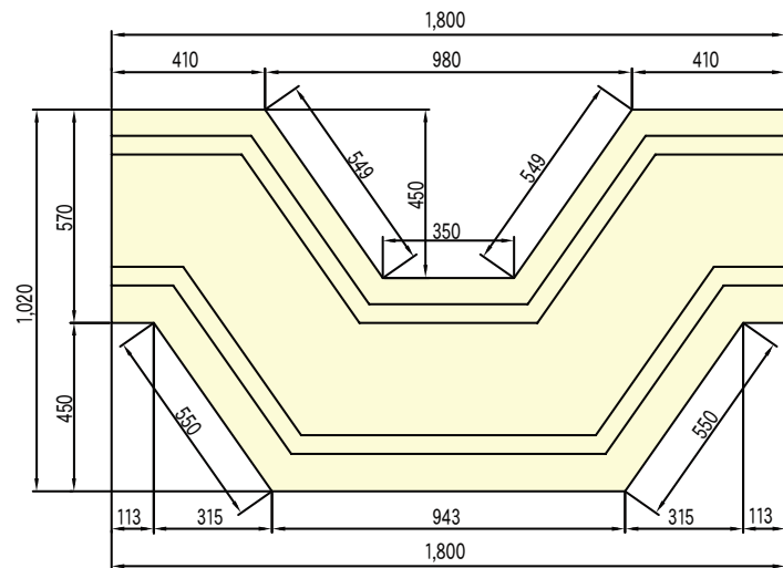
■ ロングU4-30 (電柱部) W=857kg
