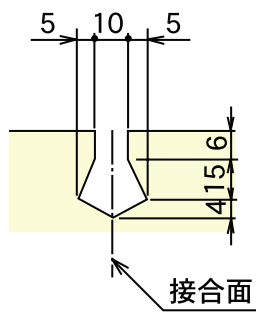
目地部詳細図
