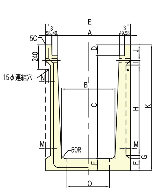
目地部詳細図
