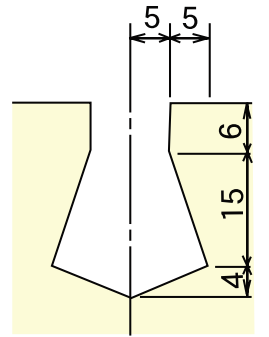
目地部詳細図
