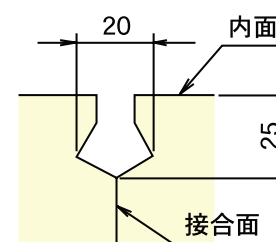
目地部詳細図 1種・3種
