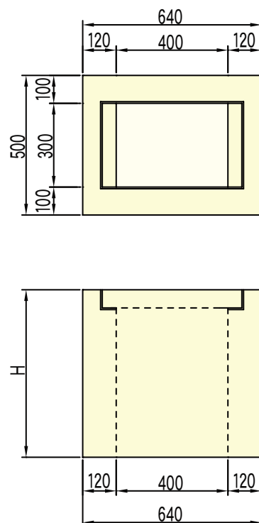
■Cドレーン縦断300用
