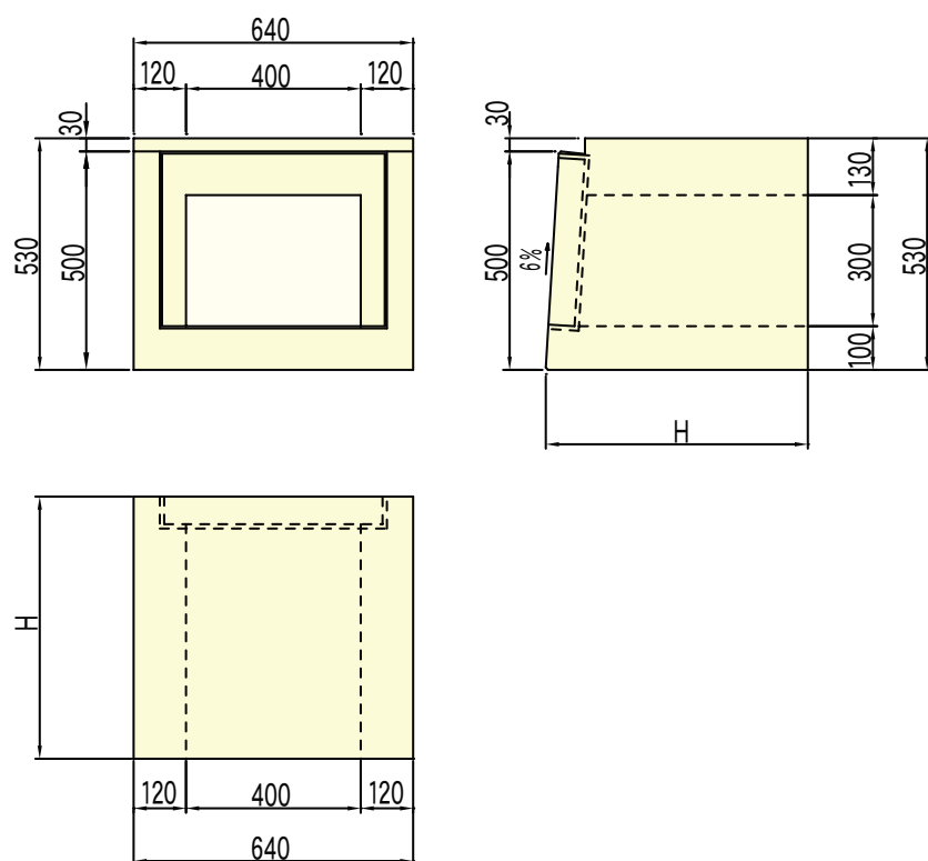
■Cドレーン街渠縦断300用 ビームボックス街渠縦断用
