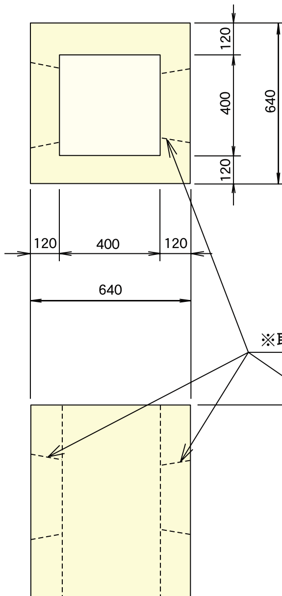
U形集水柵躯体
